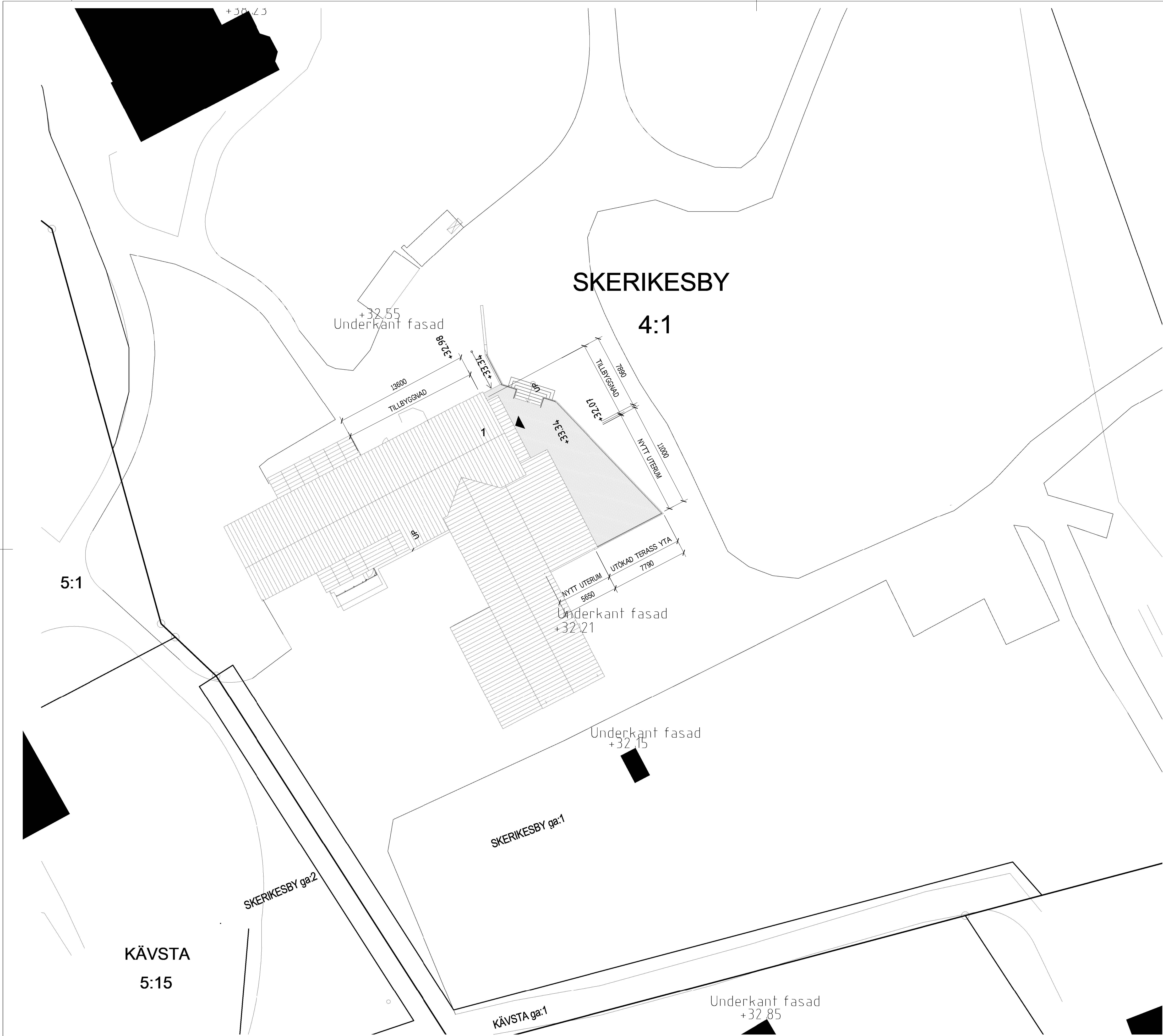
SITUATIONSPLAN SKALA 1 : 200
